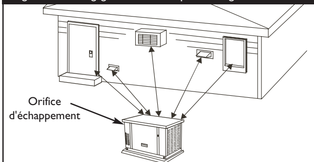
Figure 29 — Dégagement du Groupe Électrogène
